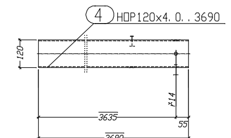
K.4 Vorderansicht
