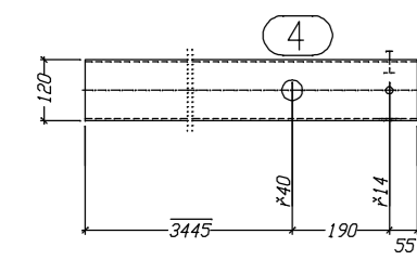
K.4 Unteransicht
