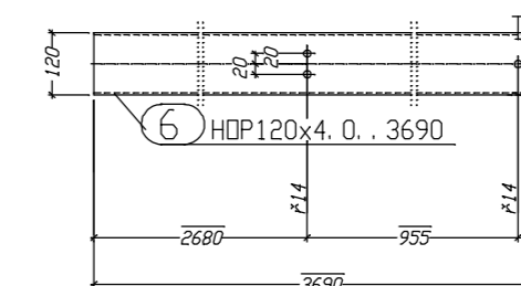
K.6 Vorderansicht
