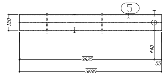
K.5 Hinteransicht
