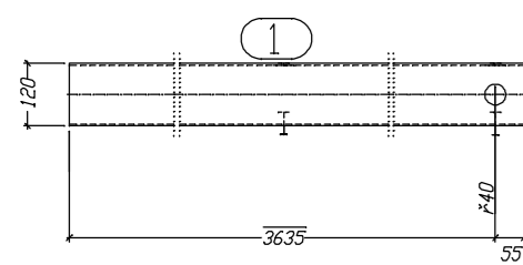
K.1 Oberansicht
