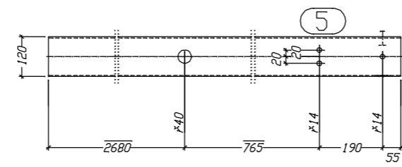
K.5 Unteransicht
