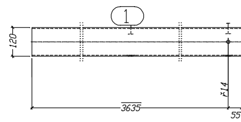
K.1 Unteransicht
