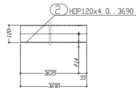
K.2 Vorderansicht
