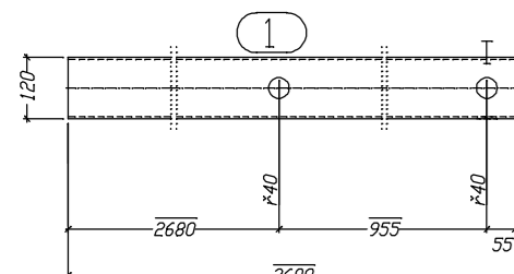
K.1 Hinteransicht
