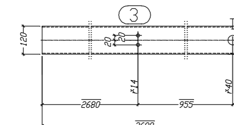
K.3 Hinteransicht
