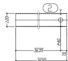
K.2 Hinteransicht
