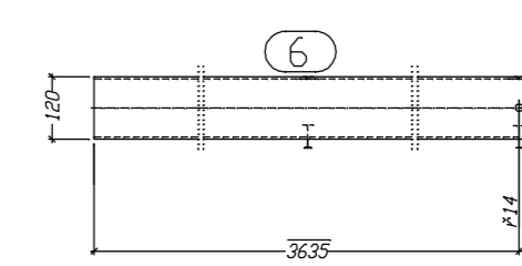
K.6 Oberansicht
