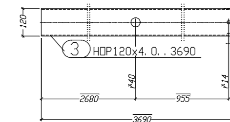
K.3 Vorderansicht
