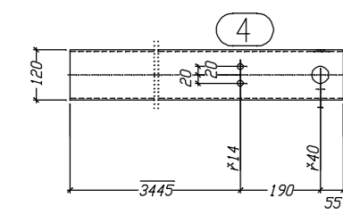
K.4 Oberansicht
