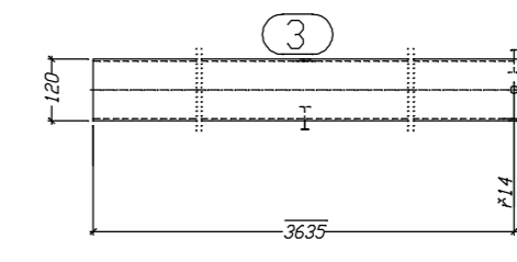
K.3 Unteransicht
