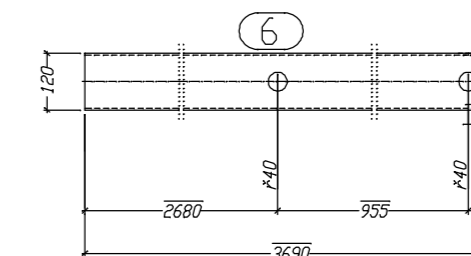
K.6 Hinteransicht
