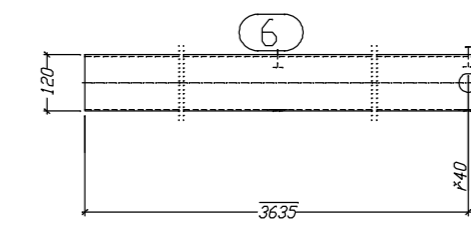
K.6 Unteransicht
