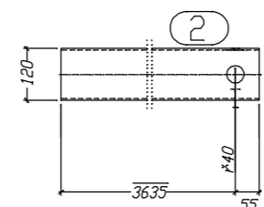
K.2 Oberansicht
