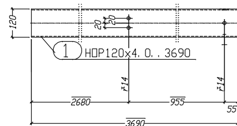
K.1 Vorderansicht
