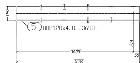
K.5 Vorderansicht
