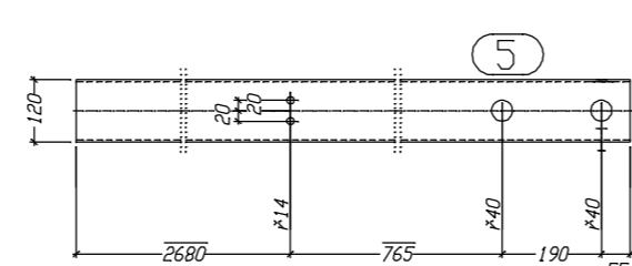
K.5 Oberansicht
